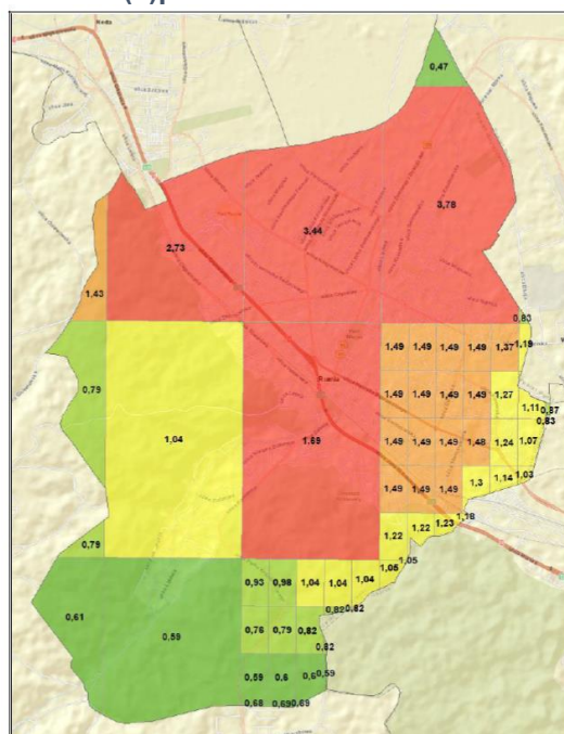
Rysunek 31. Wartości stężeń benzo(a)pirenu na terenie Rumii 94
