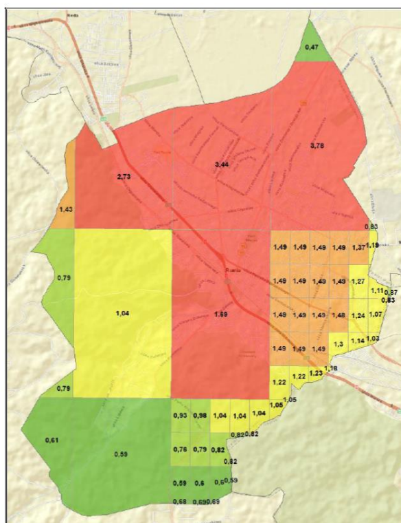
Rysunek 11. Wartości stężeń benzo(a)pirenu na terenie Rumi 38
